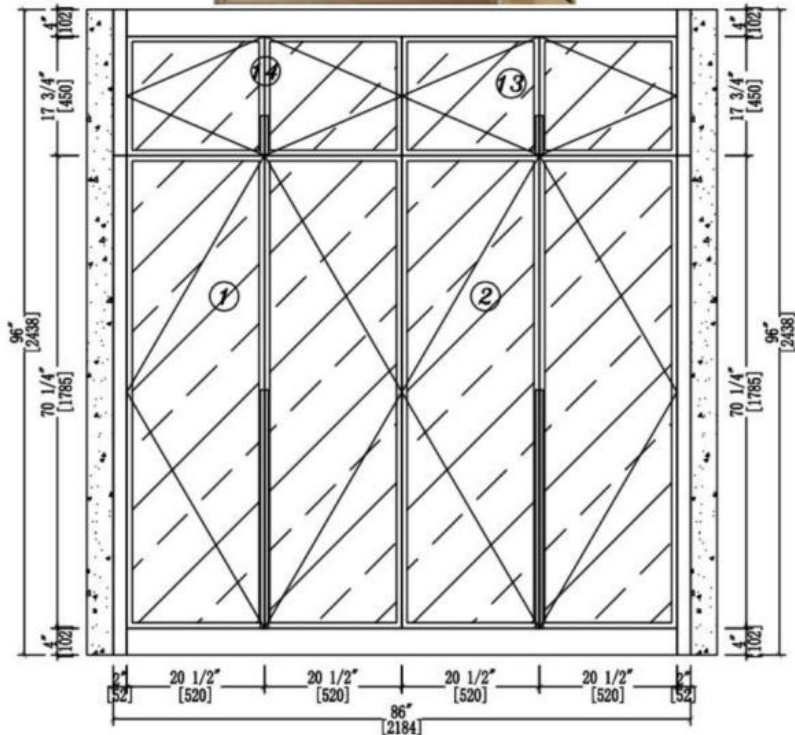
A ELEVATION
